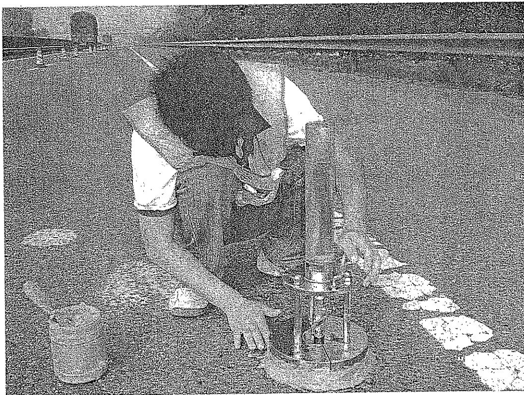
附图 1 路面渗水试验
