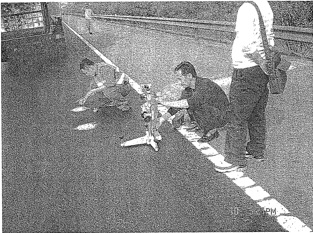
附图 3 路面抗滑性能测试
